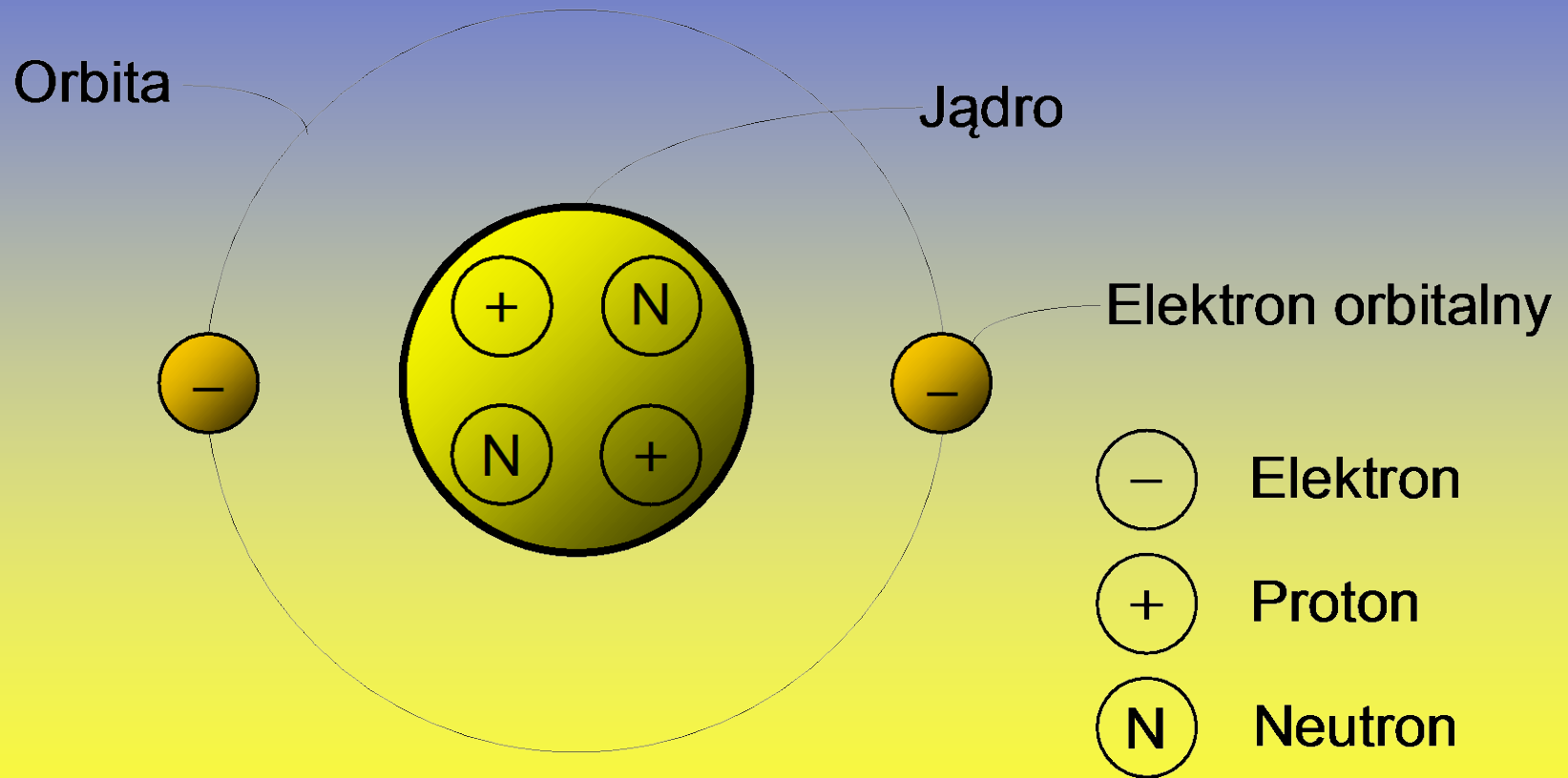
Atom helu
