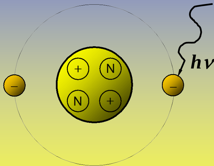
Atom niezjonizowany
