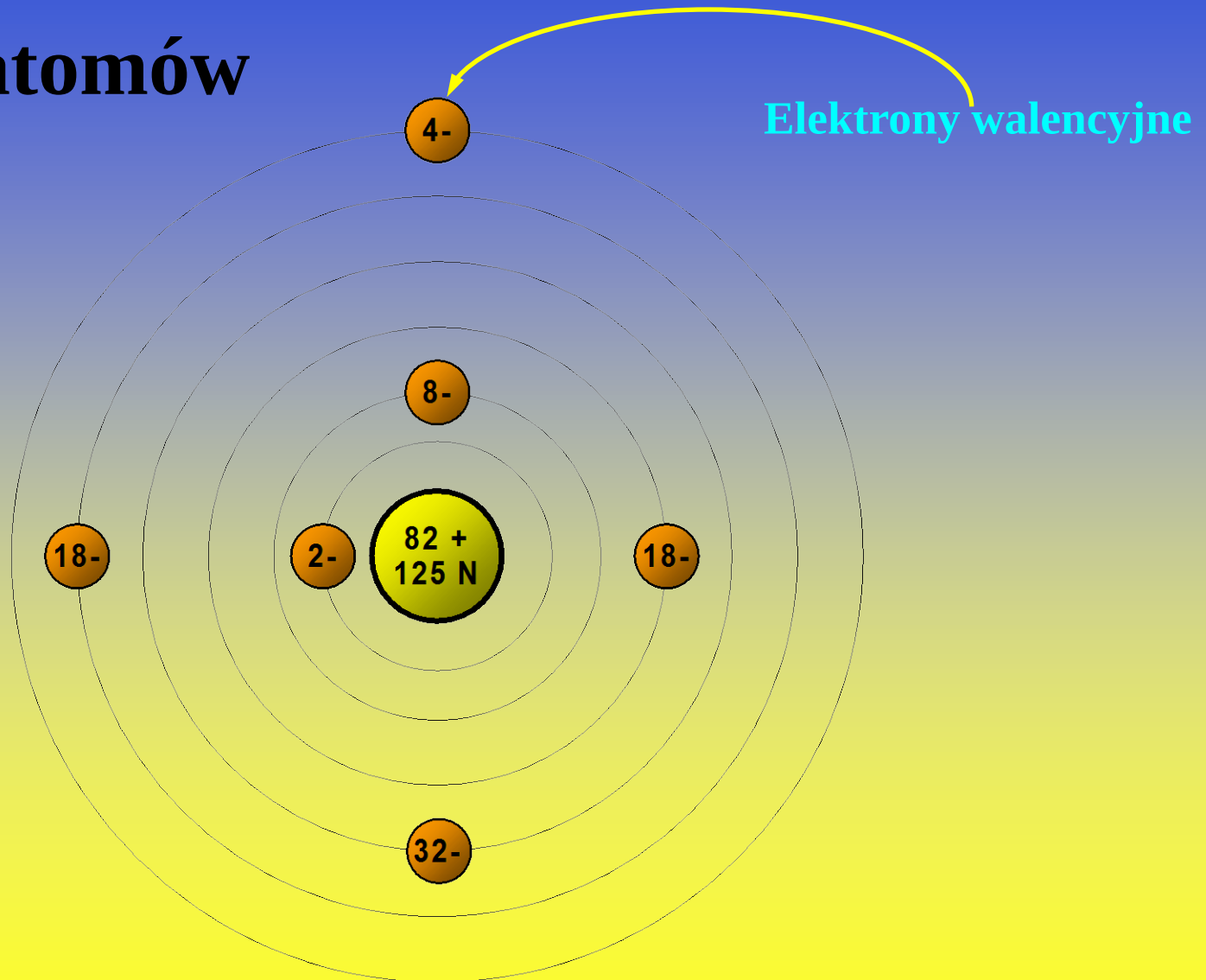
Atom ołowiu
